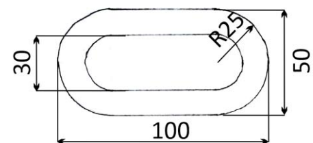
oko reťaze
